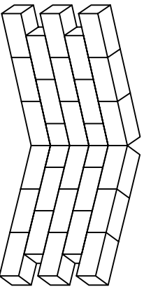
INSIDE ANGLE -NO BATTER (MSE WALL)
