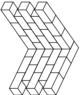
90° CORNER -NO BATTER (MSE WALL)
