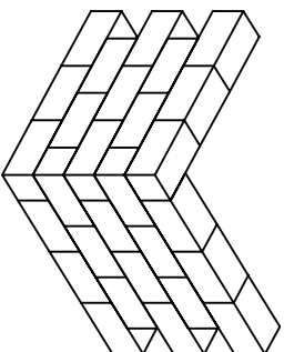
90° CORNER -NO BATTER (MSE WALL)
